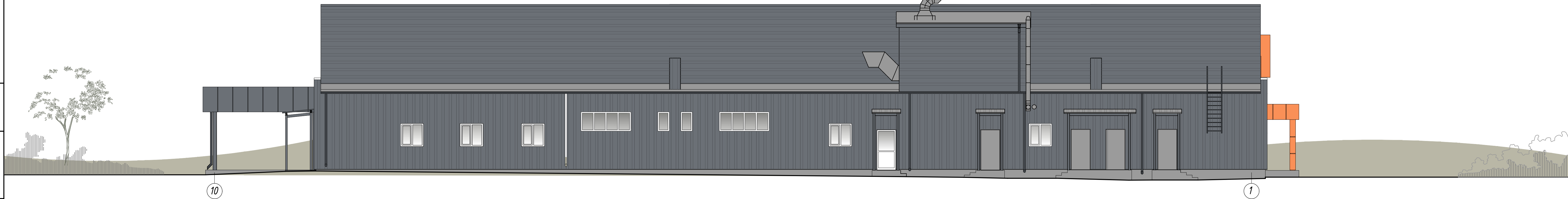
Фасад в осях 10-1
